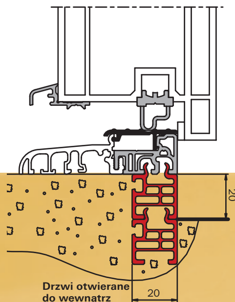
Profil poszerzający z tworzywa sztucznego KS-20
