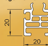
Profil poszerzający z tworzywa sztucznego KS-20
