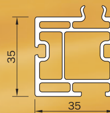
Zaślepki do profili poszerzających z tworzywa sztucznego KS-35 (możliwość skracania)
