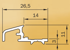
Profil odwadniający III
