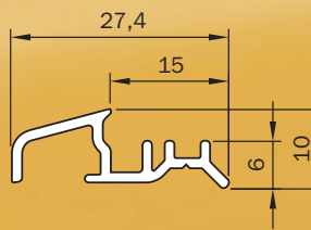
Profil odwadniający IV
