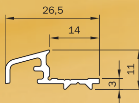
Profil odwadniający II
