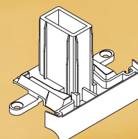
BKV 62 T BKV 70 T BKV 75 T
