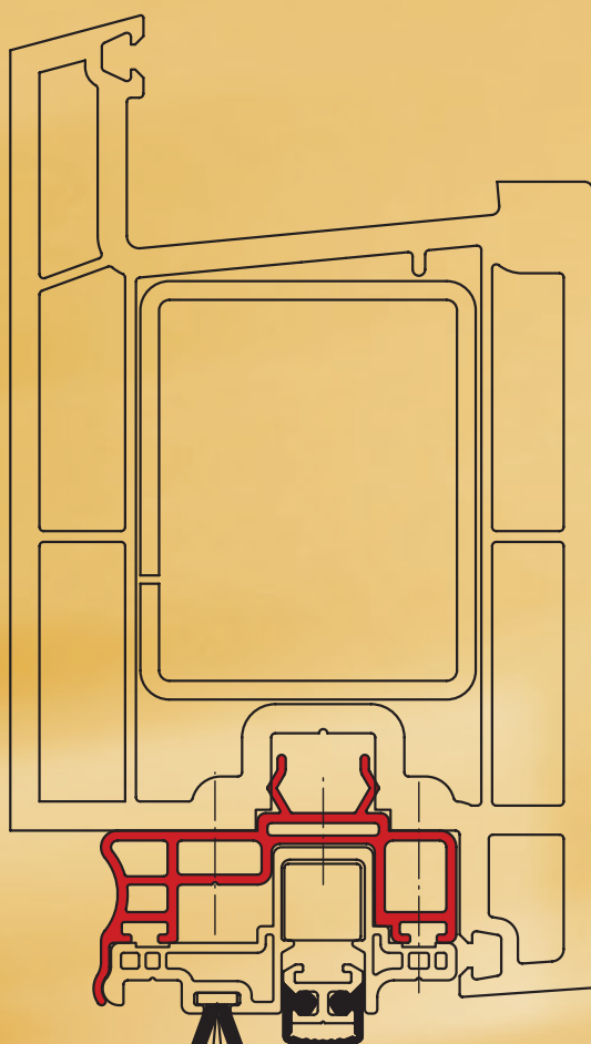
BKV – Profil dodatkowy do drzwi bezprogowych z zastosowaniem uszczelnienia Texel
