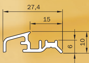
Profil odwadniający I
